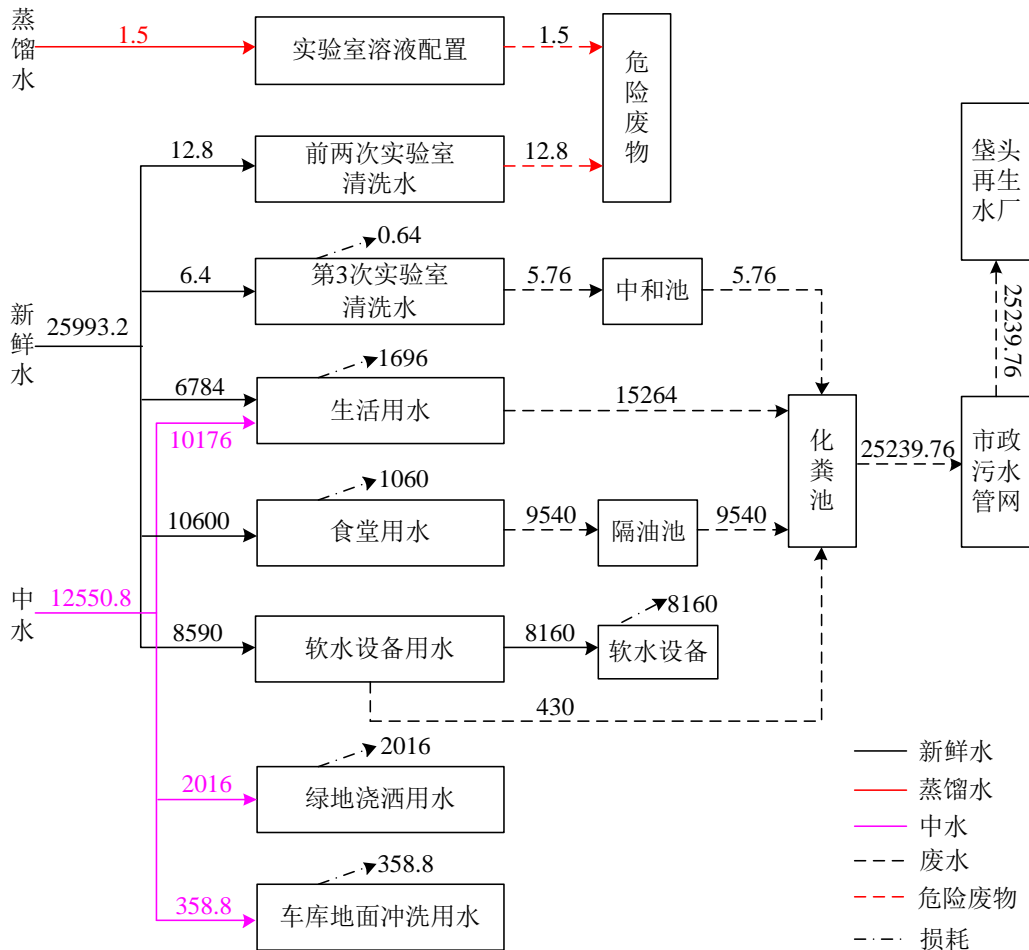
图2-1 本项目年水平衡图（单位：m³/a）
