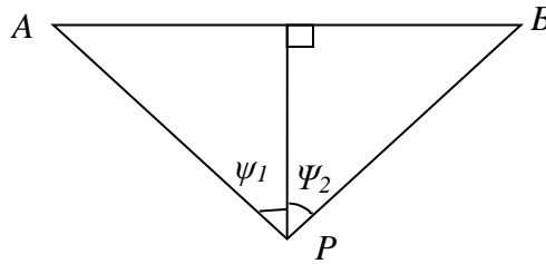
图 4-2 有限路段的修正函数，A—B 为路段，P 为预测点
