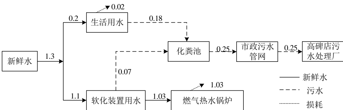
图 2-3 本项目最小日用水量平衡图 (m³/d)
