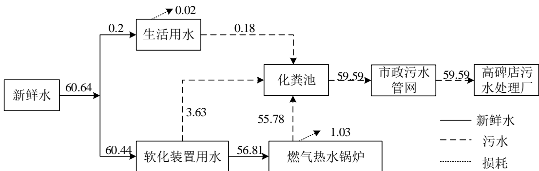
图 2-2 本项目最大日用水量平衡图 (m³/d)
