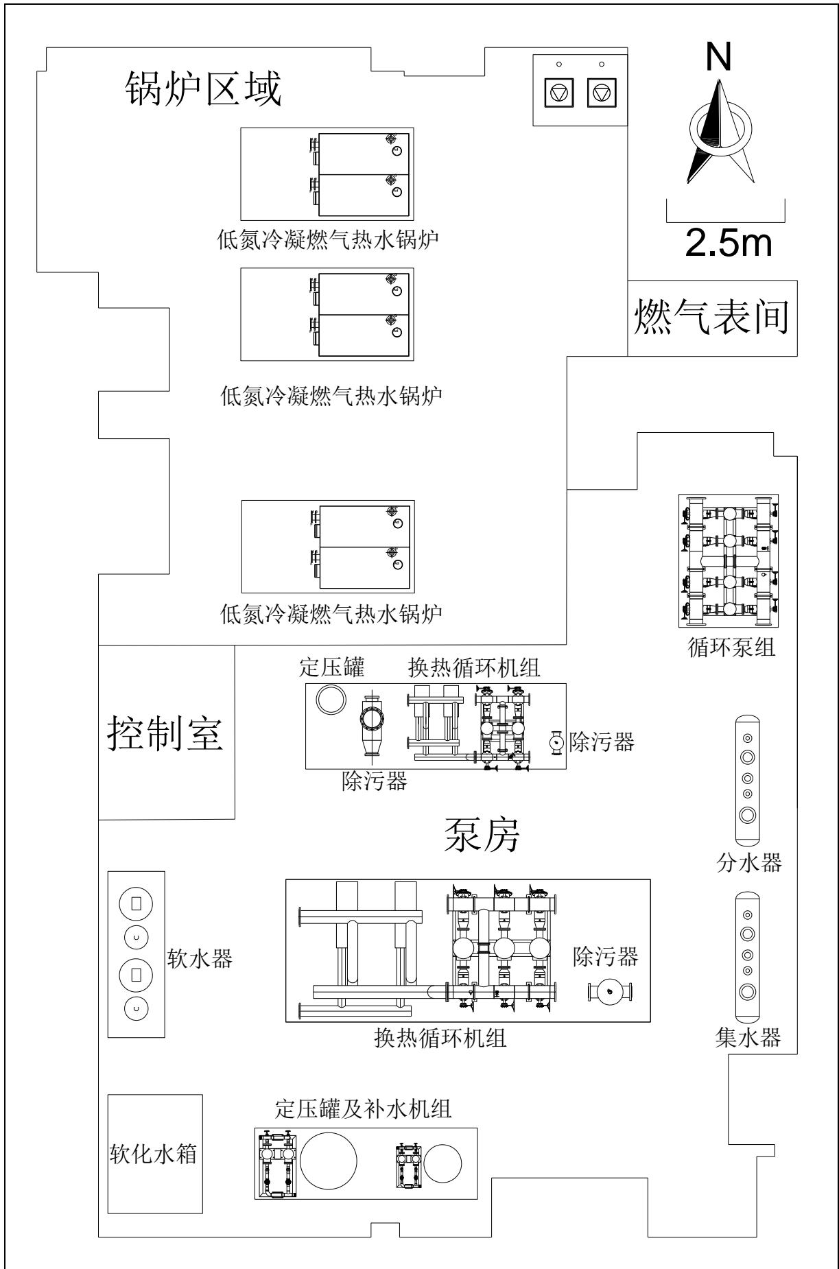
附图 4 锅炉房平面布置图
