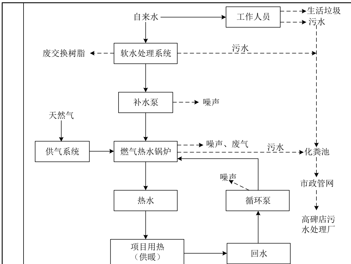
图 2-5 运营期工艺流程图
