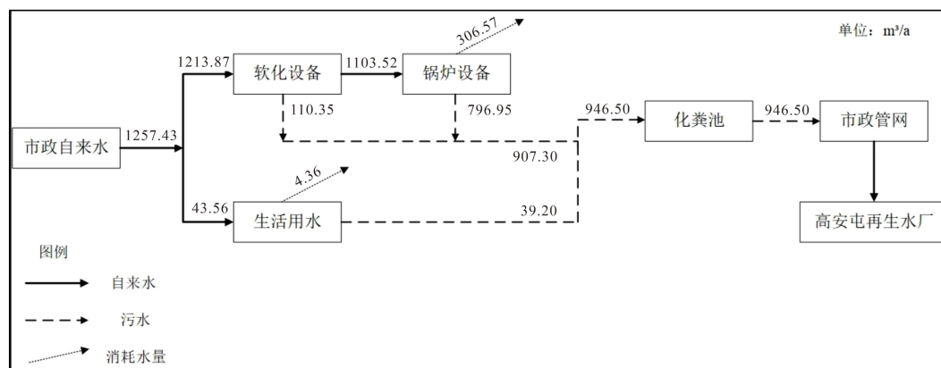
图3 本项目年水平衡图
