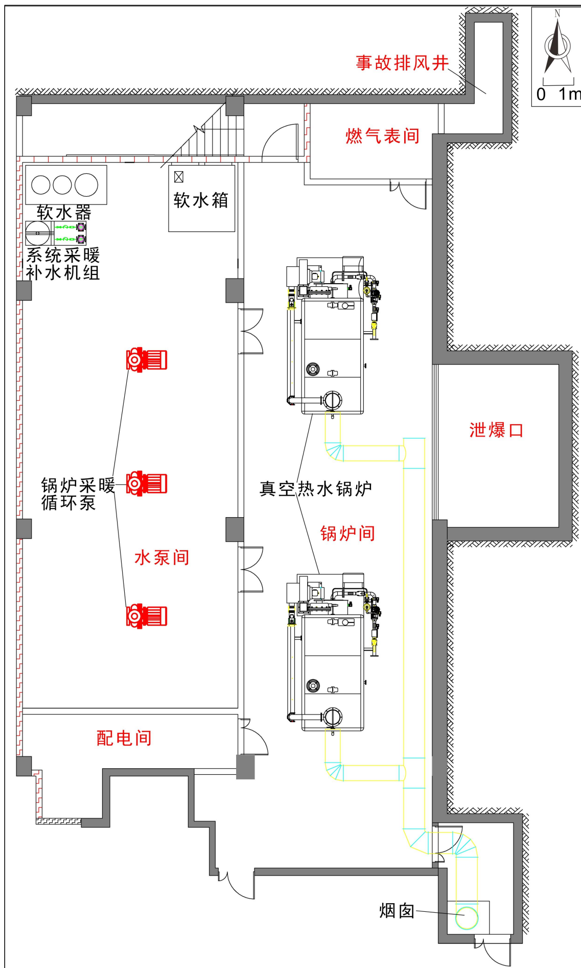
附图 4 锅炉房平面布置图
